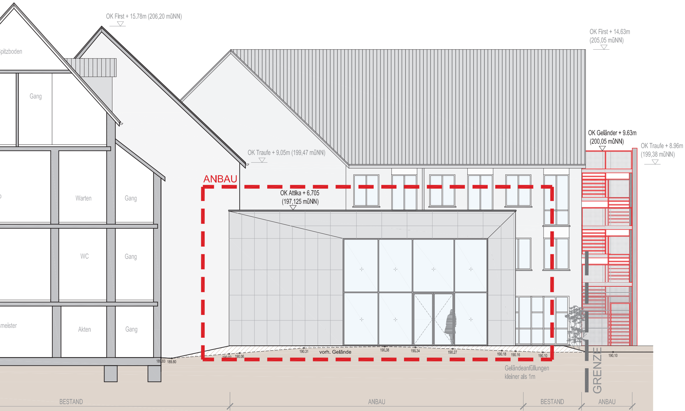
SCHNITT B-B / SÜDANSICHT
