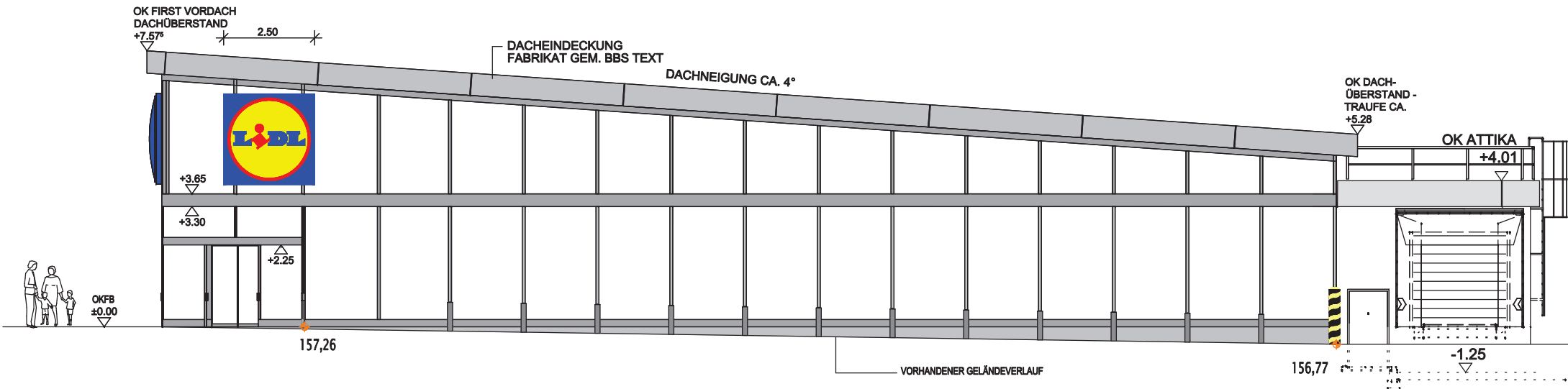
NORD-WEST ANSICHT
